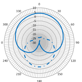
Vertical (ETSI)
