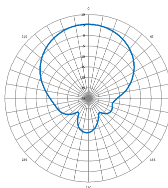
Horizontal (ETSI)
